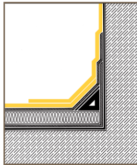
Cant Strip sur isolant avec étanchéité bicouche
